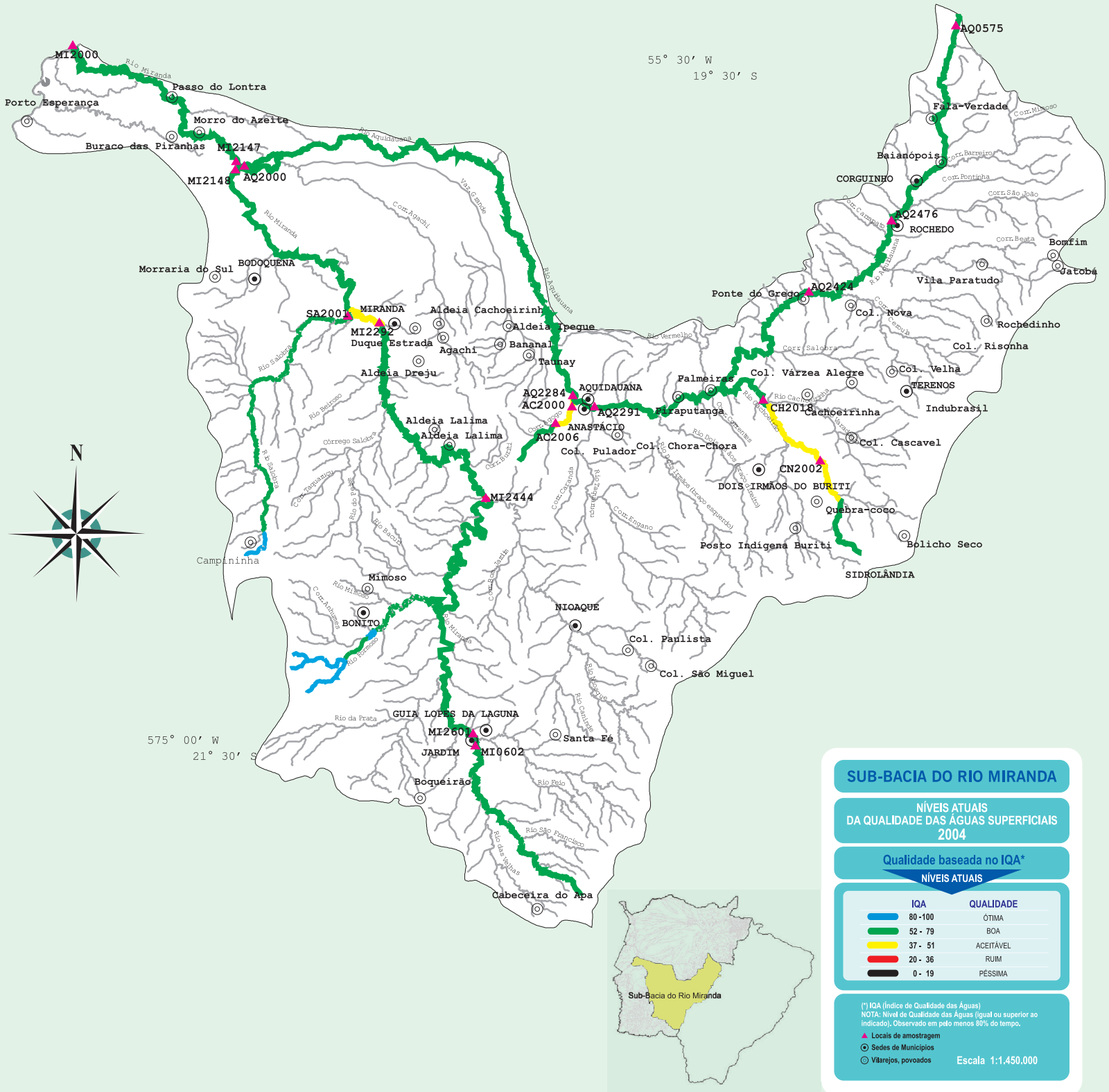
Figura 12. Níveis da qualidade das águas superficiais da sub-bacia do rio Miranda, avaliada pelo IQA, 2004.
